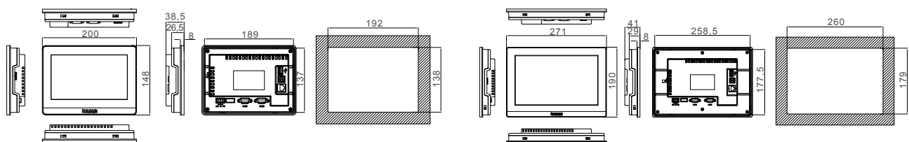
HV01-070SE / Установочный размер
